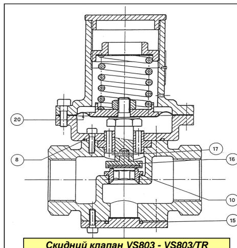
Скидний клапан VS803 - VS803/TR
