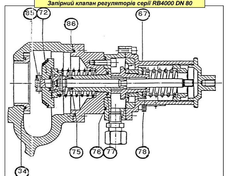
Запірний клапан регуляторів серії RB4000 DN 80
