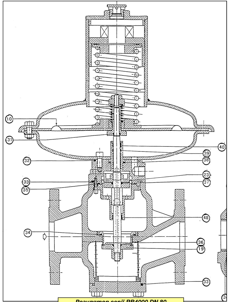
Регулятор серії RB4000 DN 80
