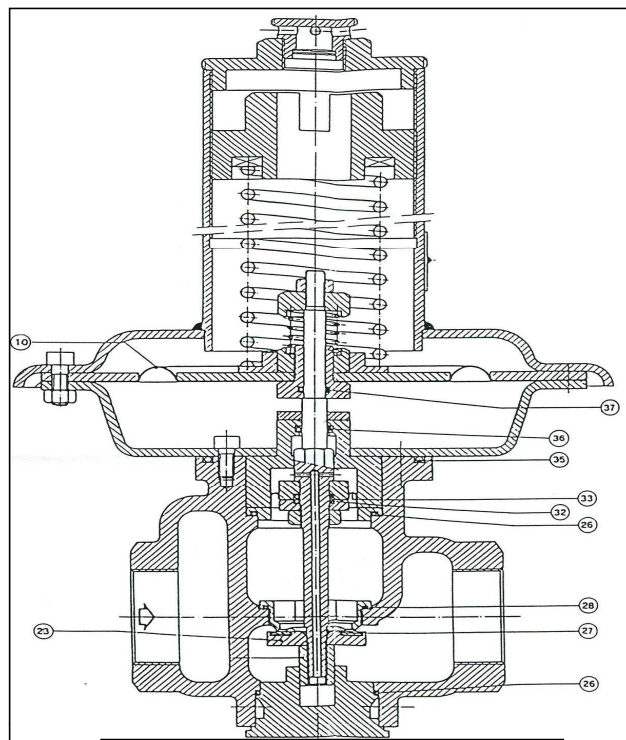
Регулятор серії RB1800 DN 1 1/2"
