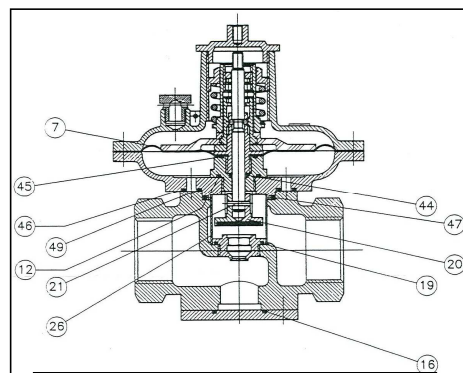
Затвірний клапан SSV8200
