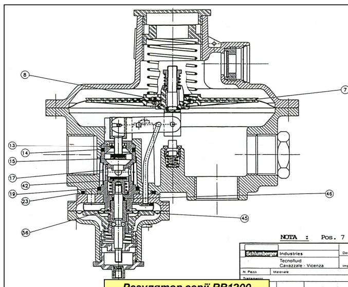
Регулятор серії RB1200
