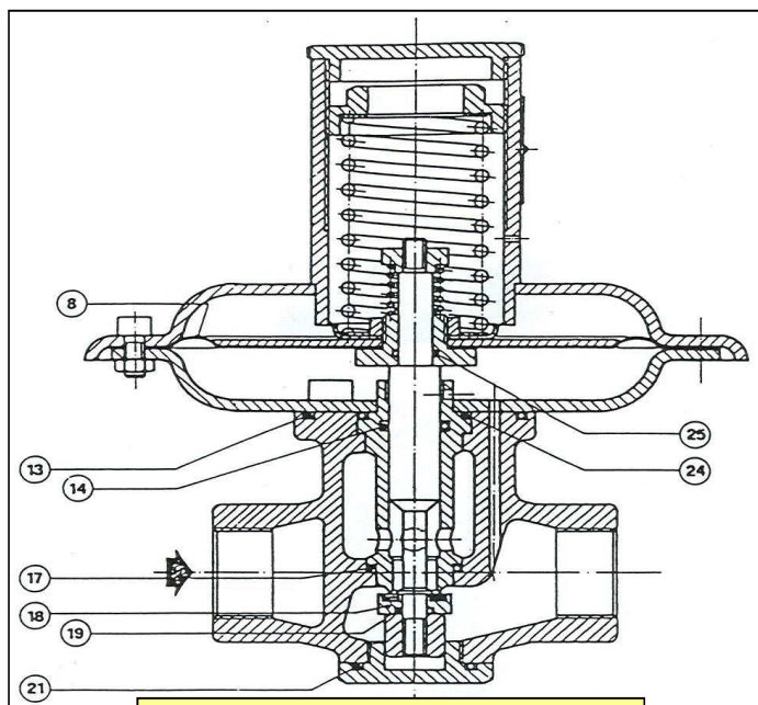
Регулятор серії RB1700 DN 3/4" - 1"
