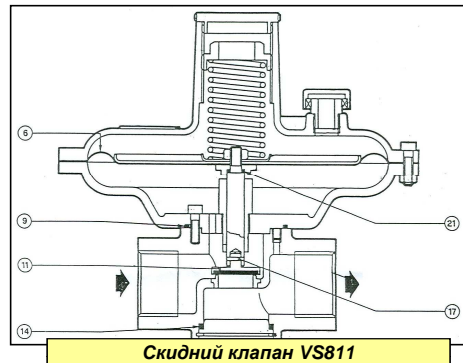
Скидний клапан VS811
