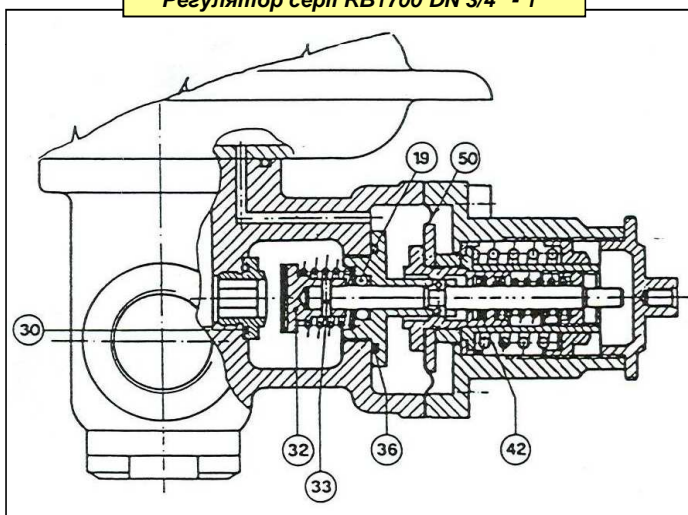
Регулятор серії RB1700 DN 3/4" - 1"
