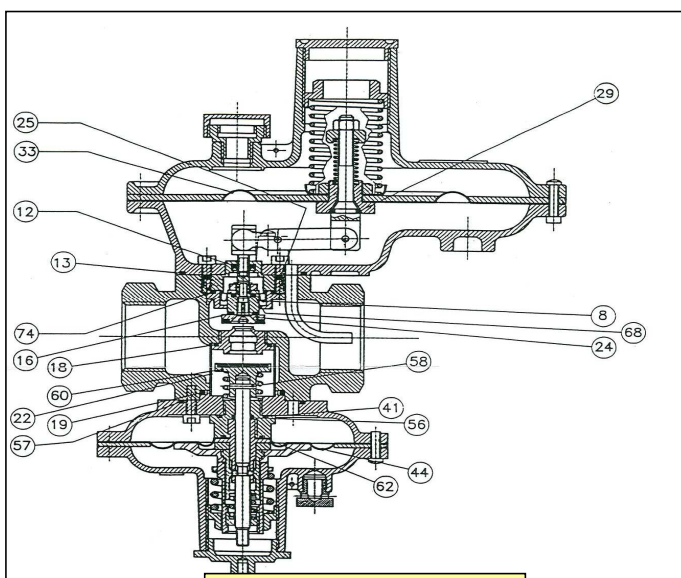
Регулятор серії RB2300-3200
