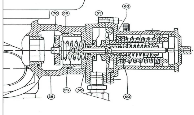
Регулятор серії RB1800 DN 1 1/2"
